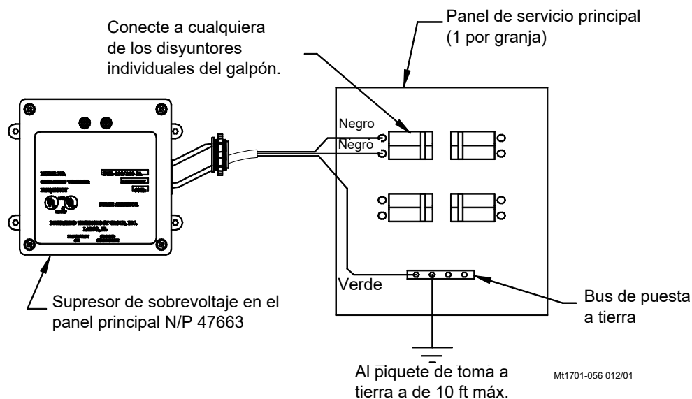
Figura 49. Alambrado del supresor de sobrevoltaje en el panel de servicio
