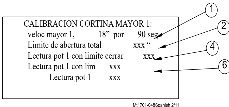
Figura 26. Calibración de potenciómetro
