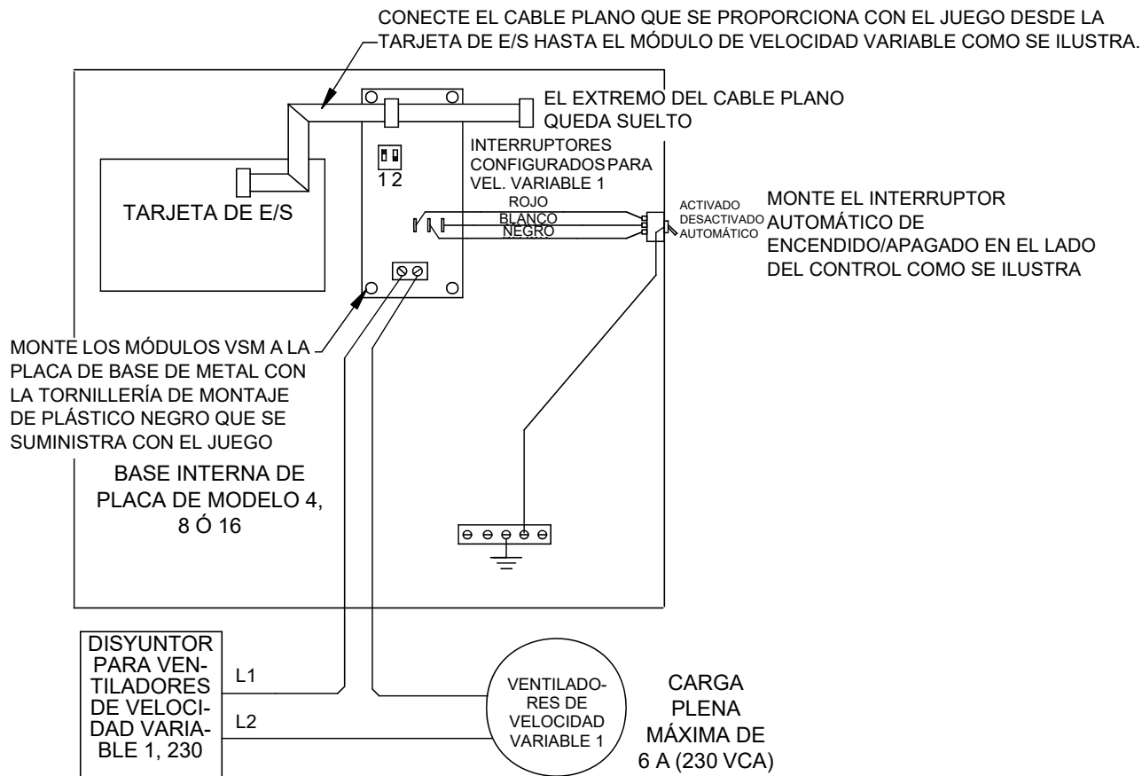
Figura 59. Alambrado del juego de velocidad variable 40729
