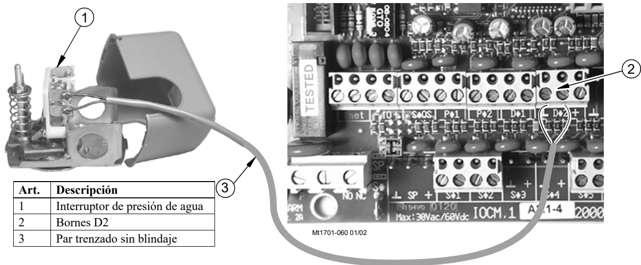
Figura 38. Alambrado del interruptor de presión de agua
