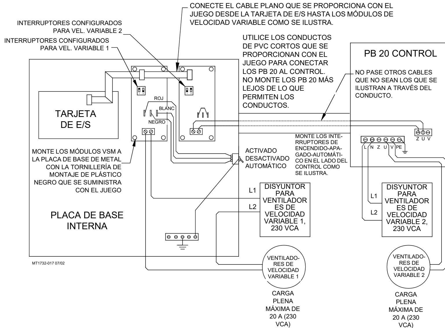
Figura 63. Alambrado del juego de velocidad variable 42523
