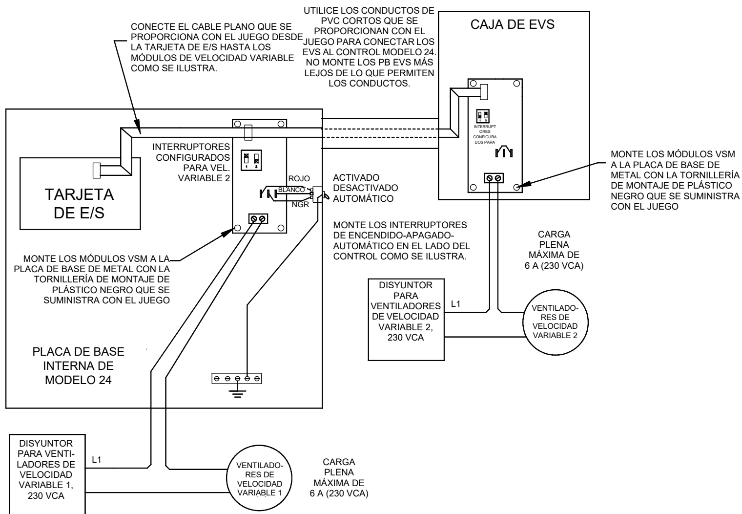
Figura 64. Alambrado del juego de velocidad variable 46568
