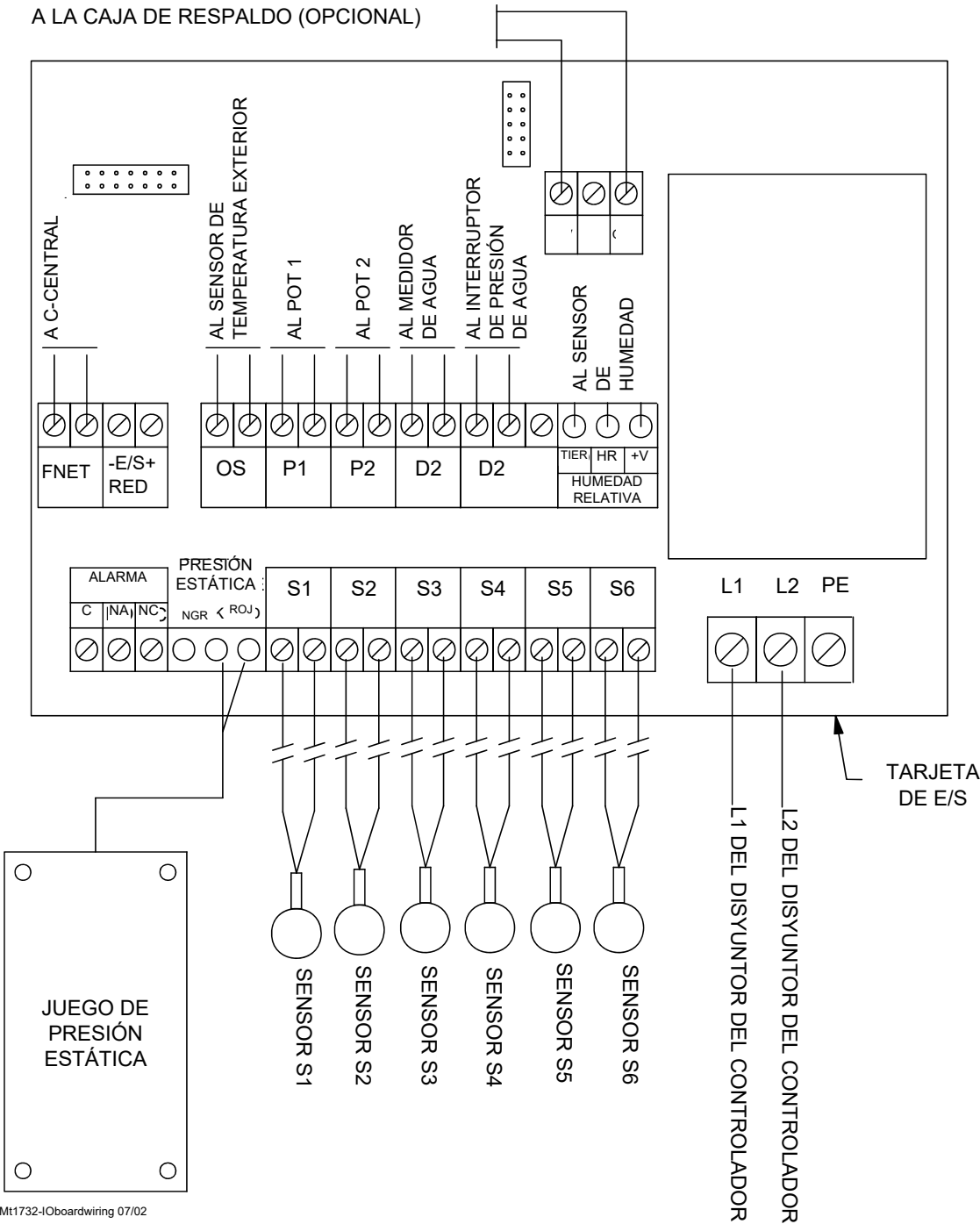
Figura 58. Alambrado de la tarjeta de E/S
