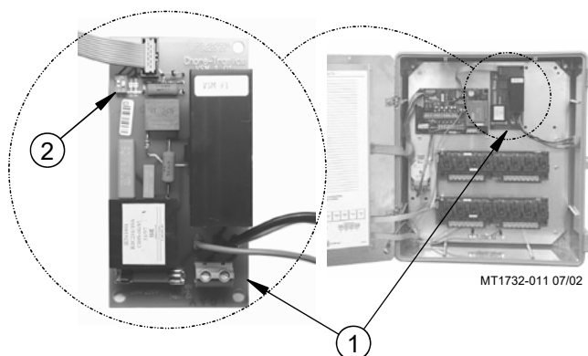
Figura 46. Interruptores DIP de velocidad variable
