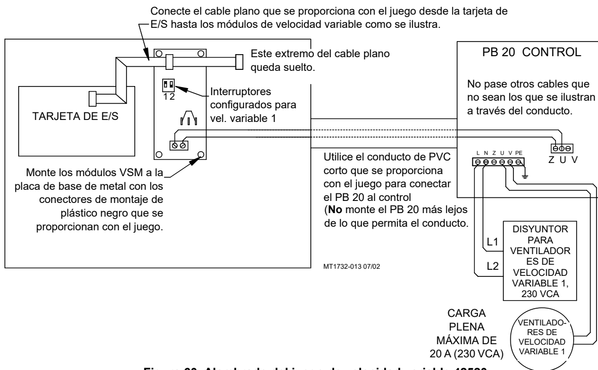
Figura 60. Alambrado del juego de velocidad variable 42520
