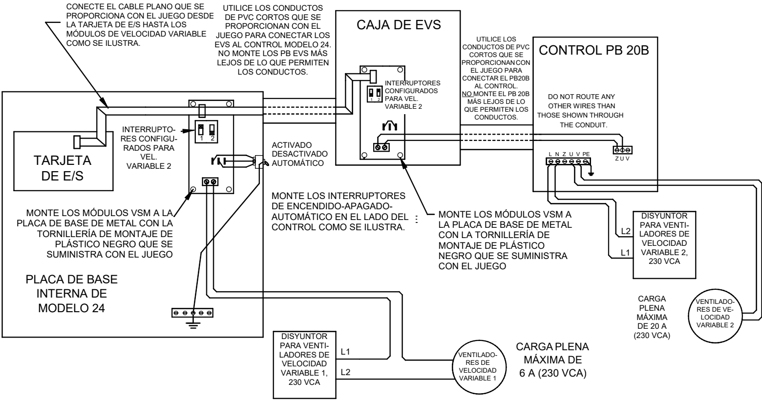
Figura 65. Alambrado del juego de velocidad variable 46569
