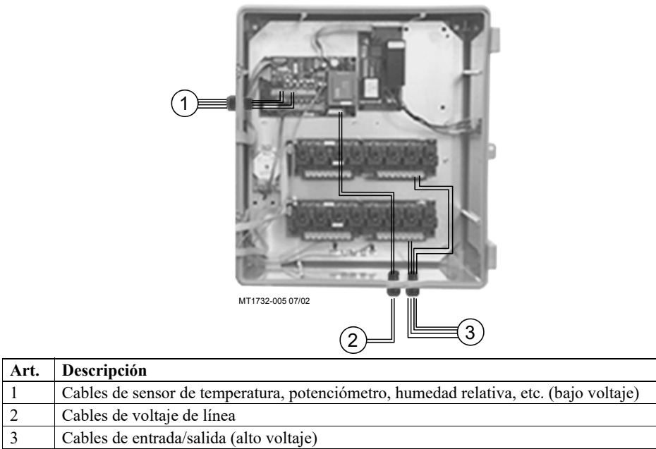
Figura 31. Colocación de cables de bajo voltaje
