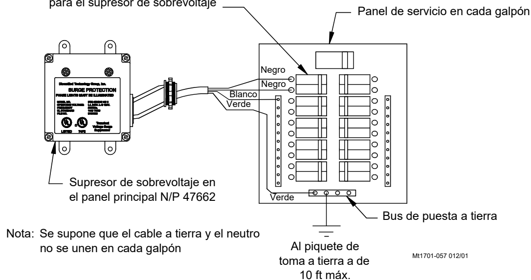
Figura 50. Alambrado del supresor de sobrevoltaje en el panel de servicio principal
