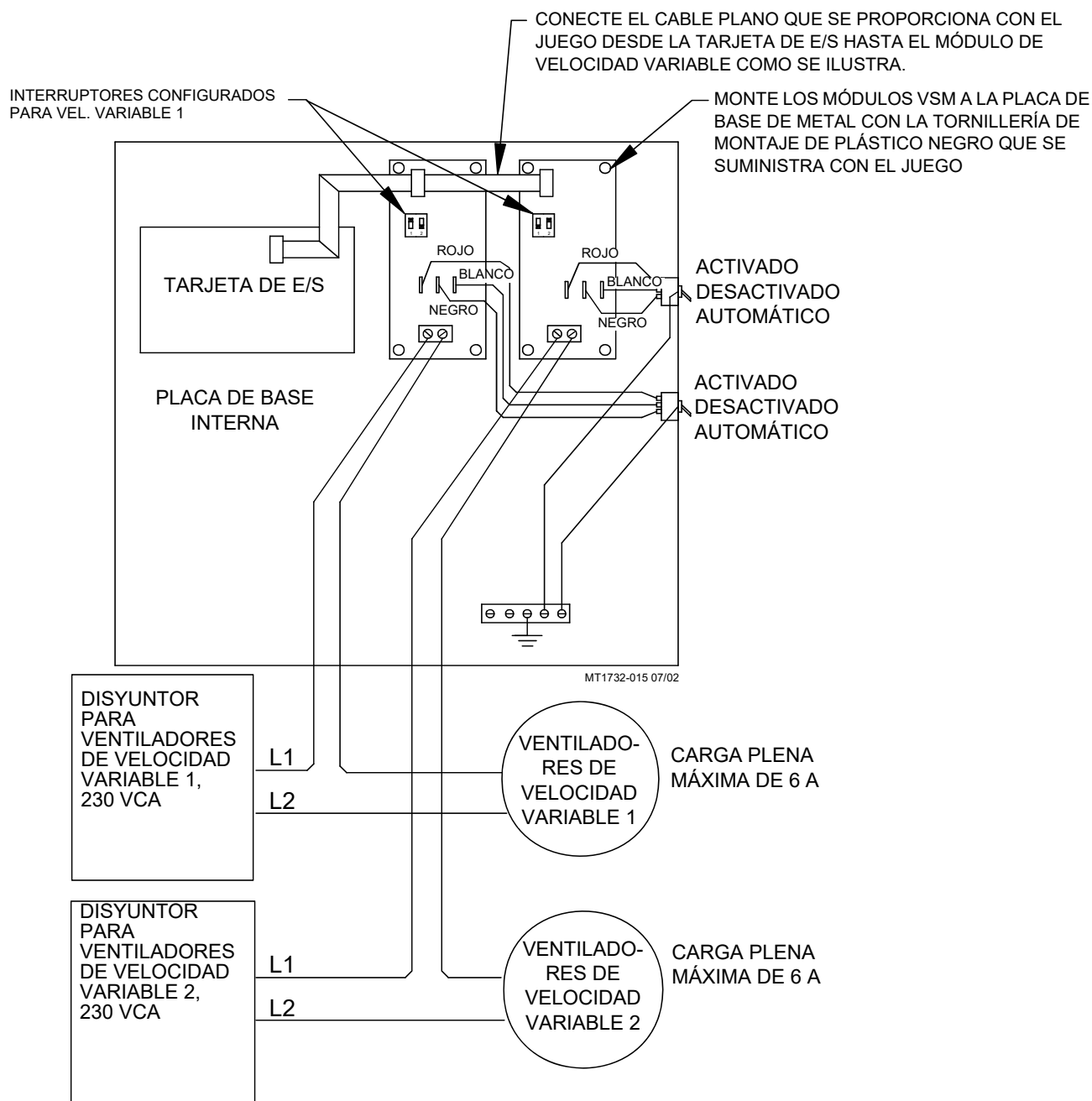
Figura 61. Alambrado del juego de velocidad variable 42521
