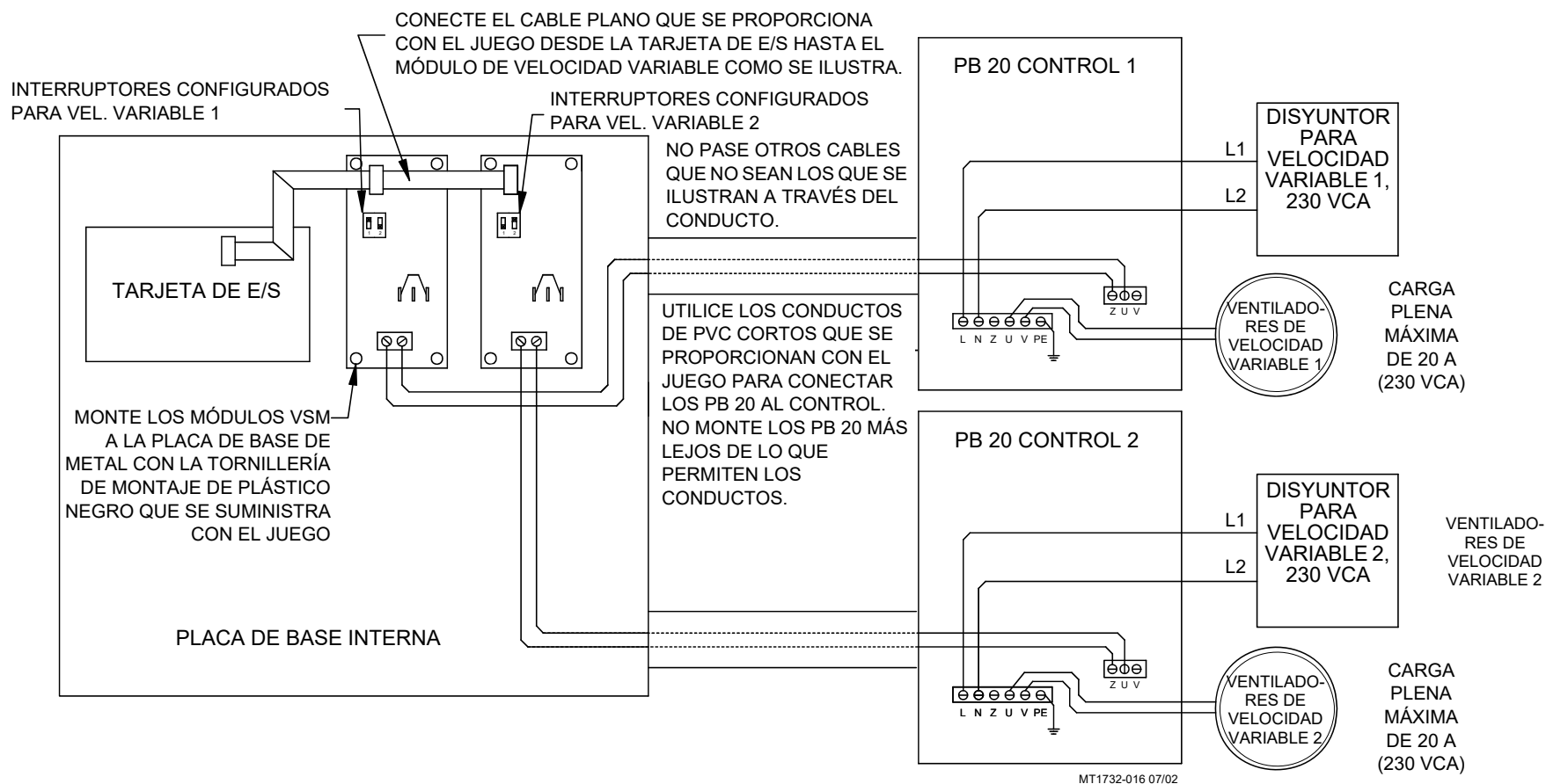
Figura 62. Alambrado del juego de velocidad variable 42522
