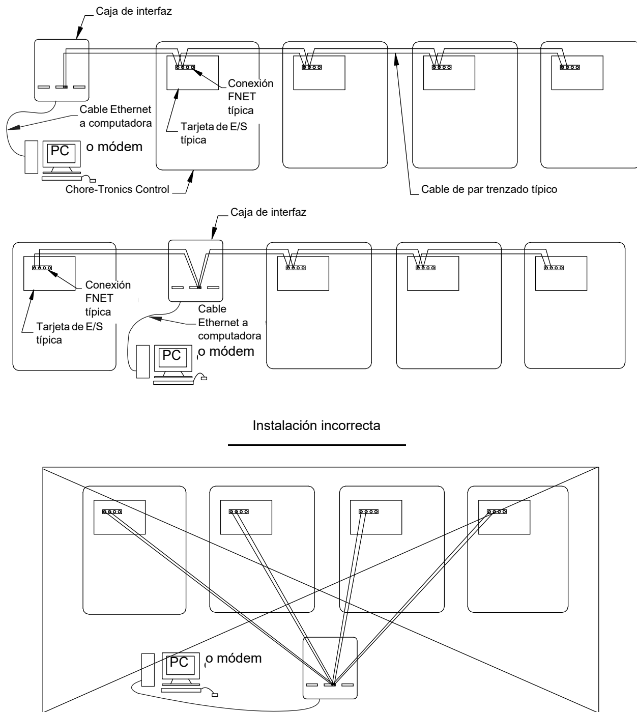
Figura 47. Conexión a una computadora
