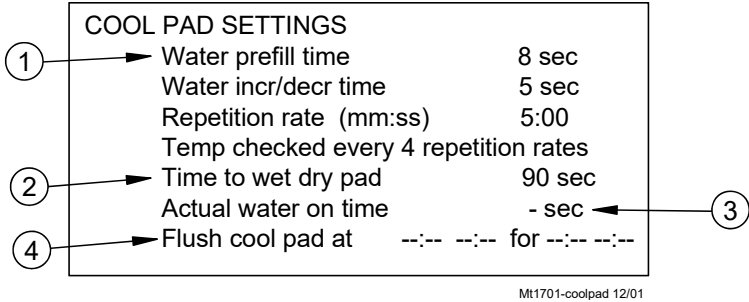
Figura 27. Configuración del panel de enfriamiento
