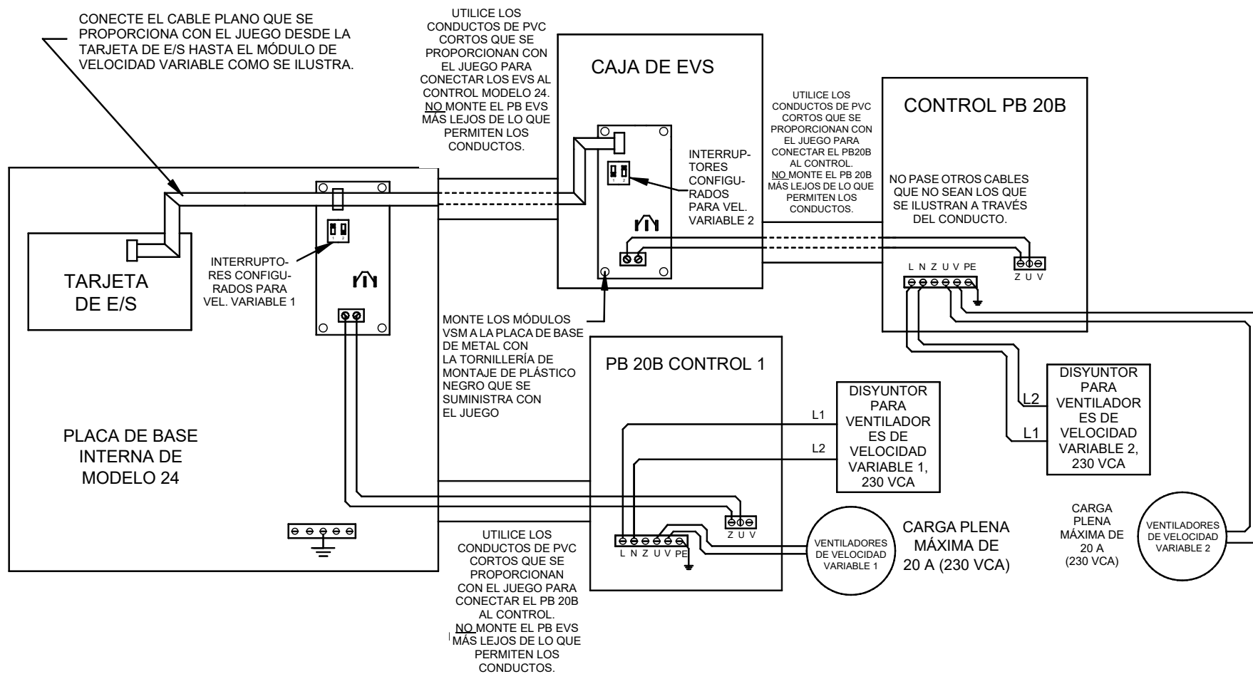
Figura 66. Alambrado del juego de velocidad variable 46570
