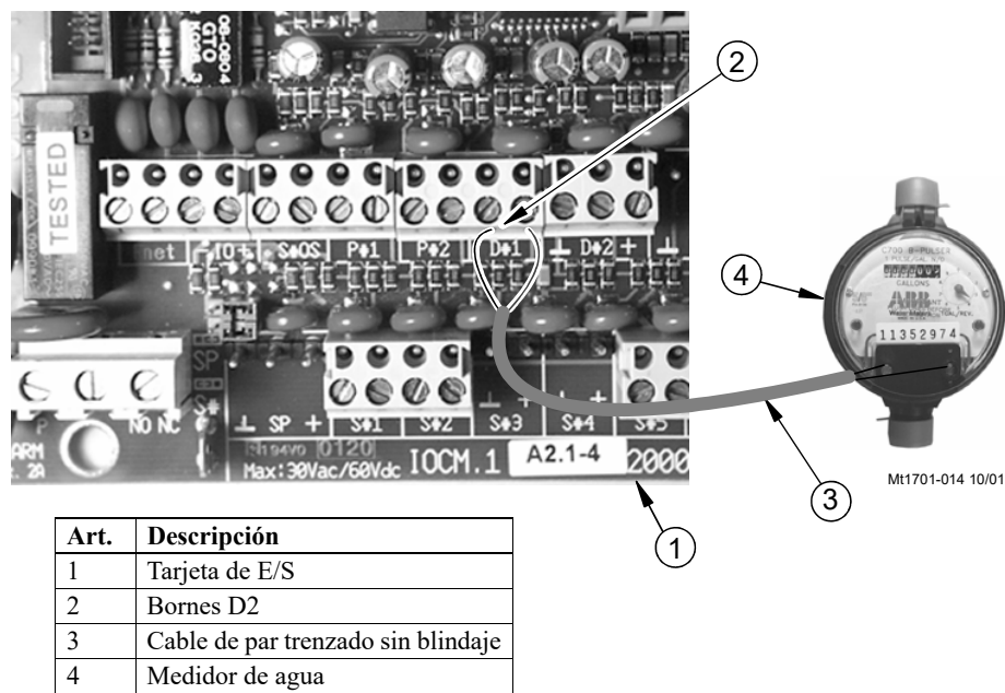
Figura 37. Medidor de agua pulsada
