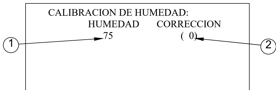
Figura 25. Sensor de humedad relativa
