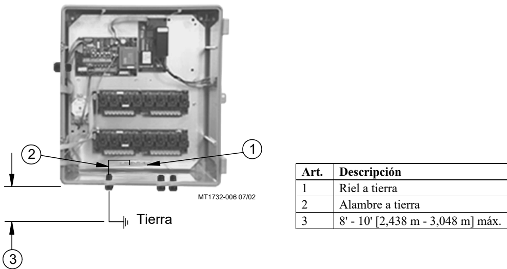
Figura 32. Colocación del cable a tierra
