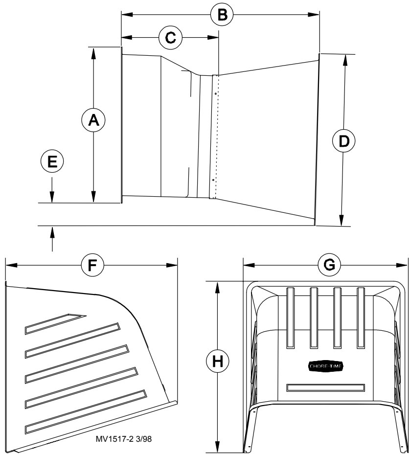
Figure 1. Fan Dimensions
