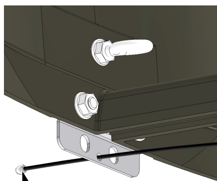
Inserte el conjunto de cable de tope de la puerta (53399) en la placa de pivote superior
