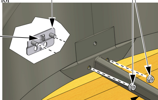
(53626) Poste en V central
