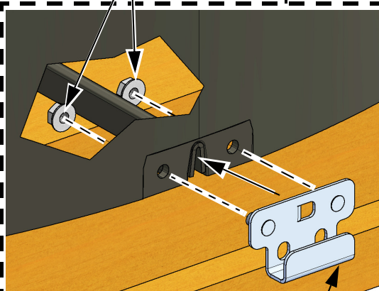
(53036) Placa de pivote inferior
