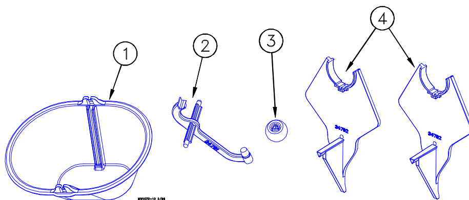
Figure 1: Mini Drinker Components
