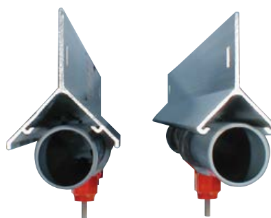
Dostępne są dwa rodzaje profili – wzmacniony (po lewej) lub standardowy.
