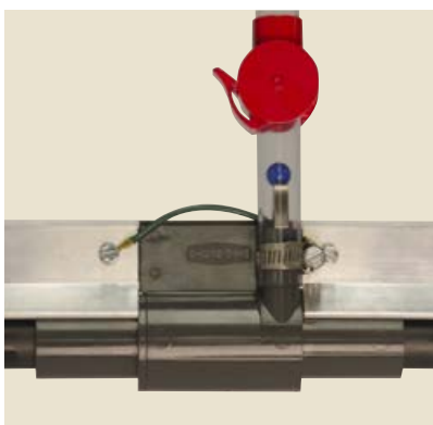
Compensador de desnivel facilita el manejo de grandes columnas de agua debido a la pendiente del piso.
