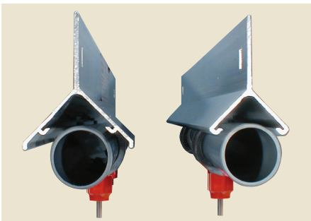
Hay dos opciones de canales de soporte disponibles: resistente (izquierda) y estándar.
