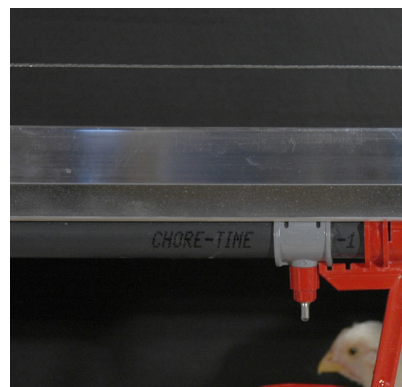
La coupelle de récupération est disponible en option pour les systèmes à haut débit et à très haut débit.
