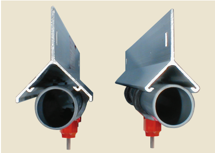
Deux options de profilés de support sont disponibles : robuste (à gauche) ou standard.
