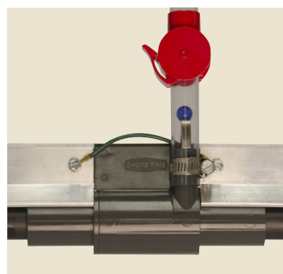
Le compensateur de pente facilite la gestion de la pression de la colonne d'eau due à l'inclinaison du sol.
