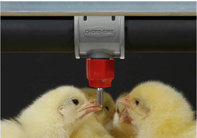
La pipette pour poulets de chair de Chore-Time est facile à déclencher par les oiseaux dès le premier jour pour une conversion alimentaire optimale en phase de démarrage.
