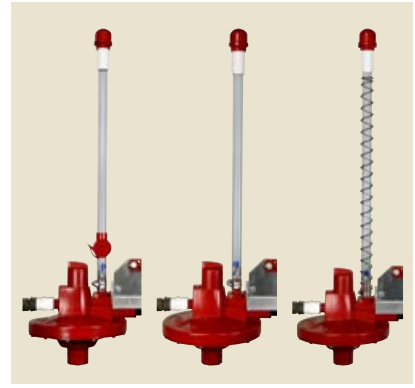
Ontluchtingsbuisopties (vanaf links): inklapbaar, vast, flexibel.
