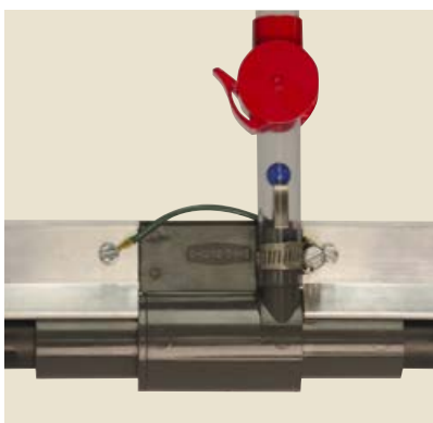
Compensatorul de pantă facilitează gestionarea volumului crescut al apei din coloana de apă care apare din cauza pantei podelei.
