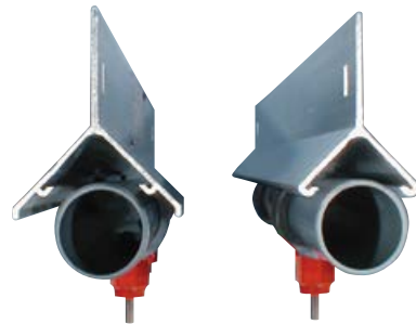
Zwei Profilloptionen sind erhältlich, hochbelastbar (links) oder Standard
