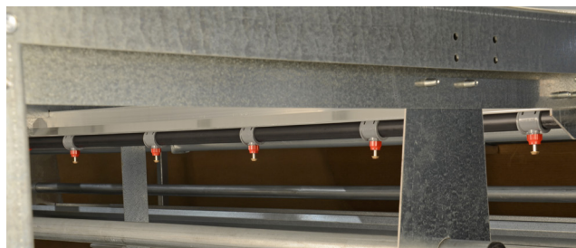
Auswahl an Chore-Time-Nippeltränkesystem ohne (Bild oben) oder mit Wasserauffangschalen (Bild unten).
