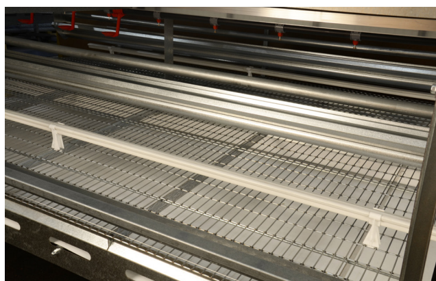
Kotbänder auf jeder Ebene halten das System stets sauber und trocken.
