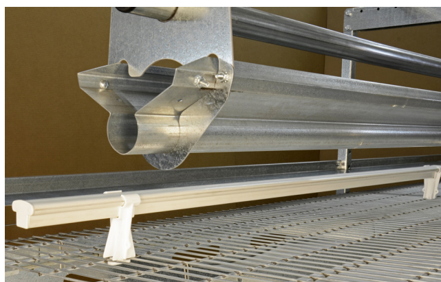
VIKER® TRADITION™ Volierensystem mit Sitzstange und Seitenansicht des ULTRAFLO®-Futtersystems.
